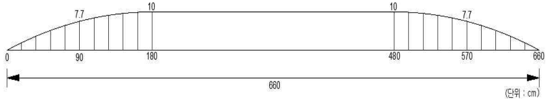
<그림 5> 어린이보호구역 전용 과속방지턱 설치 규격
